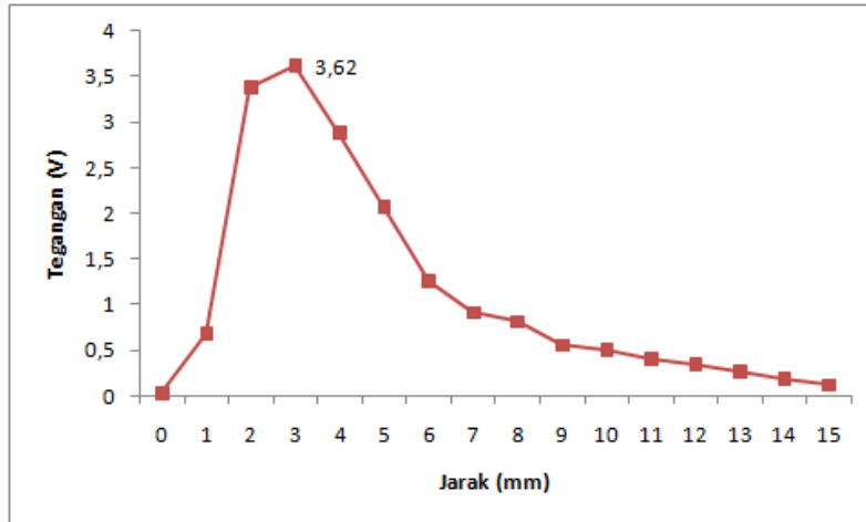
Gambar 2. Hubungan antara jarak pengukuran dan tegangan yang dihasilkan pada pengukuran pergeseran mikro
