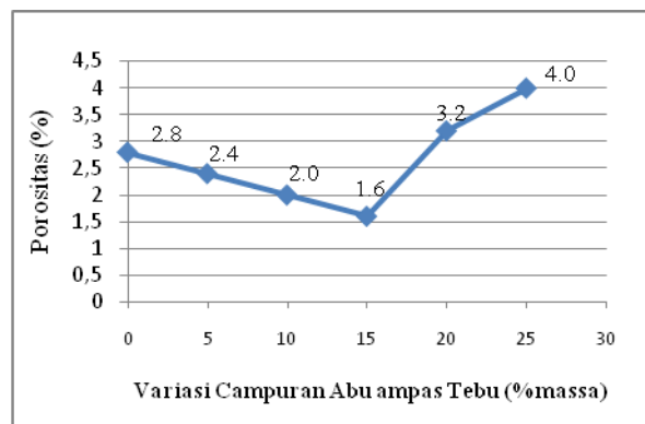
Gambar 7 Grafik porositas terhadap variasi campuran abu ampas tebu
