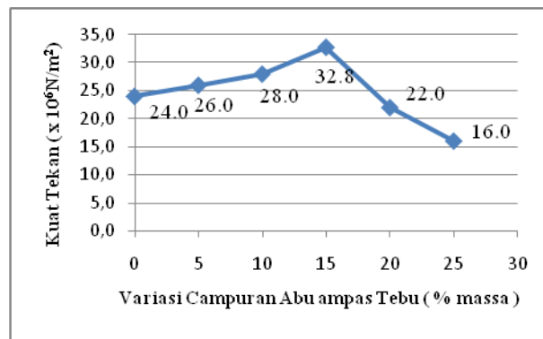
Gambar 1 Kuat tekan terhadap variasi campuran abu ampas tebu
