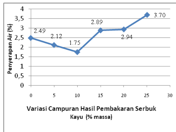
Gambar 10 Penyerapan air terhadap variasi campuran hasil pembakaran serbuk kayu
