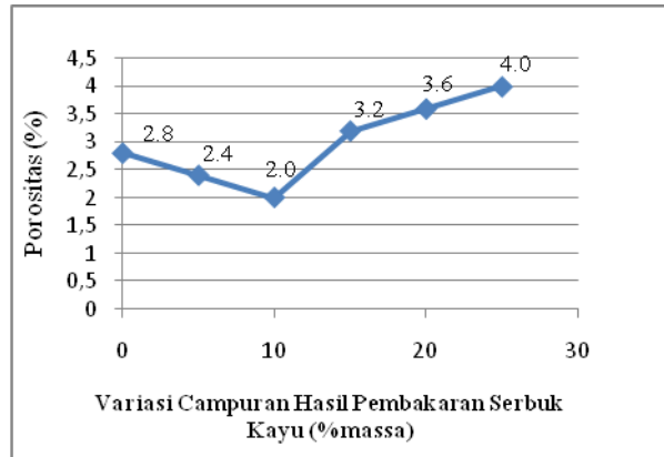
Gambar 8 Porositas terhadap variasi campuran hasil pembakaran serbuk kayu
