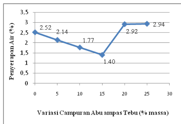
Gambar 9 Penyerapan air terhadap variasi campuran abu ampas tebu
