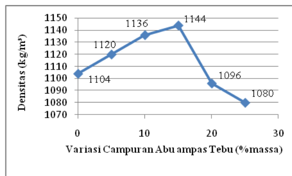
Gambar 5 Densitas terhadap variasi campuran abu ampas tebu
