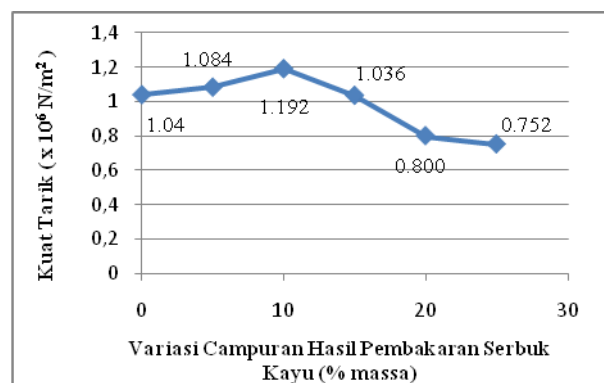
Gambar 4 Kuat tarik terhadap variasi campuran hasil pembakaran serbuk kayu
