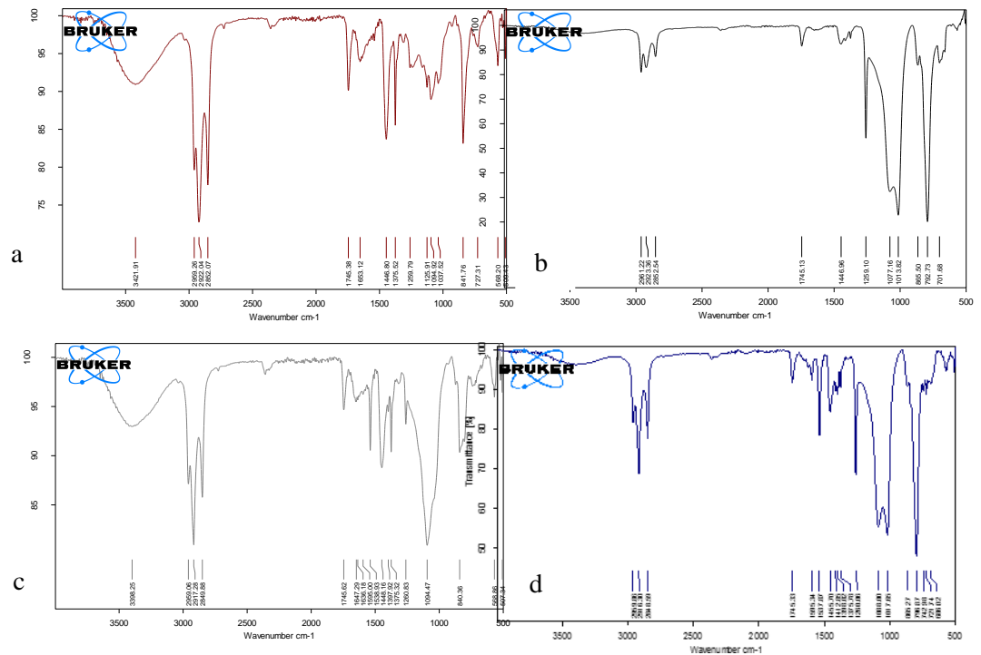
Gambar 1 Hasil Karakterisasi Transmittansi sampel kontrol 100% lateks (a), sampel dengan Karet Komposit Lateks 50% dan Silikon50% (b), sampel dengan Karet Komposit Lateks75% dan Silikon25% (c) dan sampel dengan Karet Komposit Silikon 100% (d)
