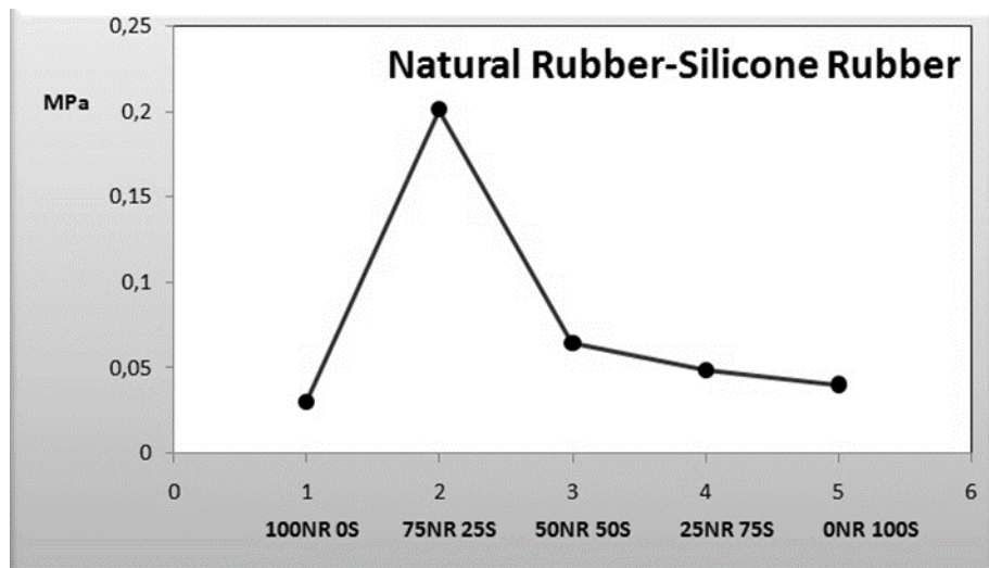
Gambar 2 Hasil Pengujian Modulus Young Sampel
